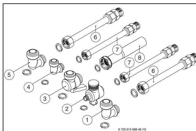
Fig. 16 Accessorio raccordi di collegamento nr. 1151 per GVS T 16/24/28-3.../GVM T...
