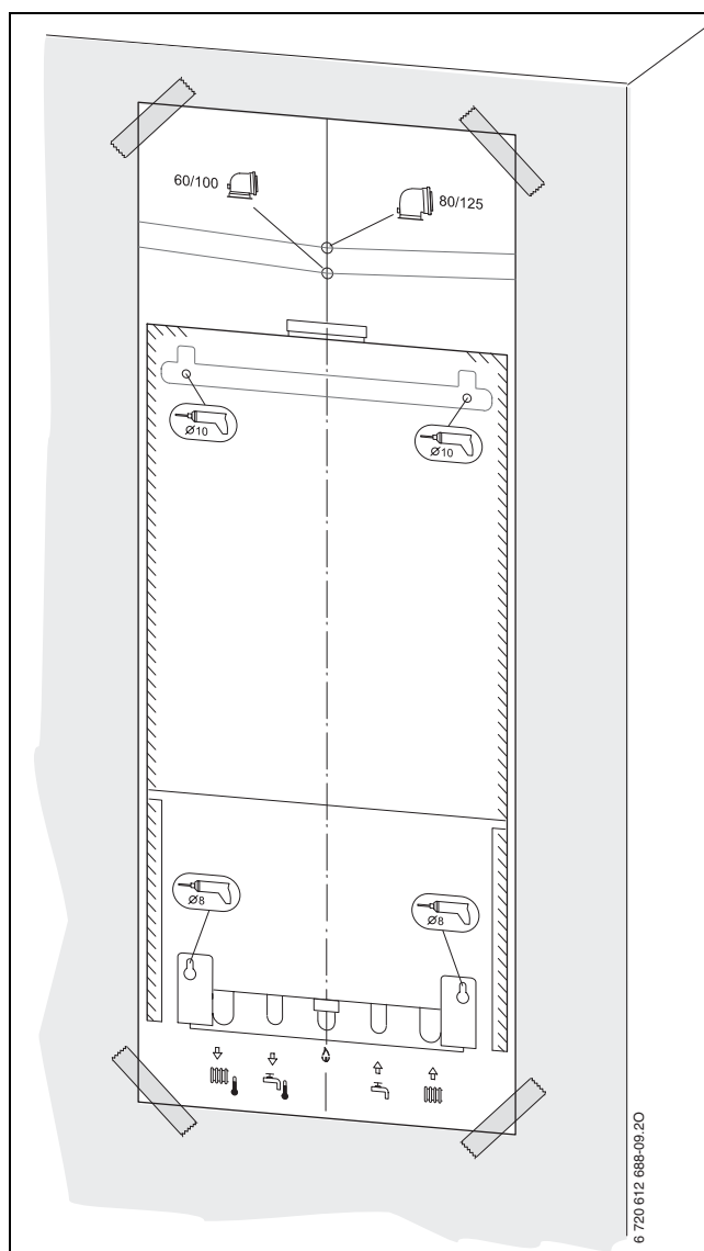
Fig. 12 Dima di preinstallazione
