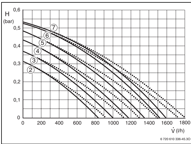
Fig. 47 Diagramma delle curve caratteristiche/velocità del circolatore
