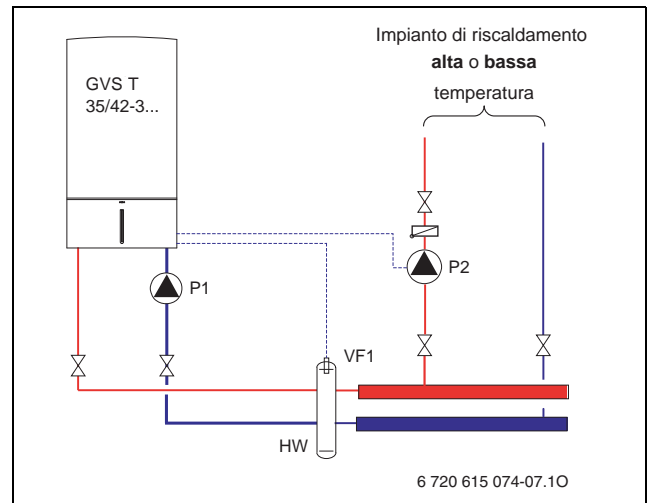
Fig. 48 Esempio d'installazione circolatore aggiuntivo
