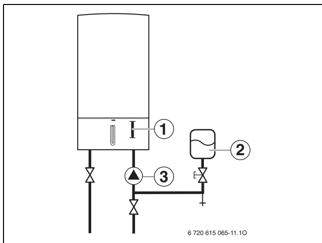
Fig. 10 Esempio installativo di accessori idraulici per GVS T 35/42-3...
