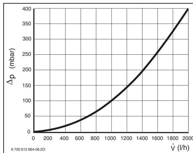
Fig. 11 Perdita di pressione per modelli GVS T 35/42-3...
