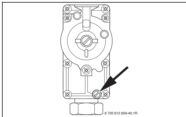
Fig. 53 Presa pressione presso gruppo gas
